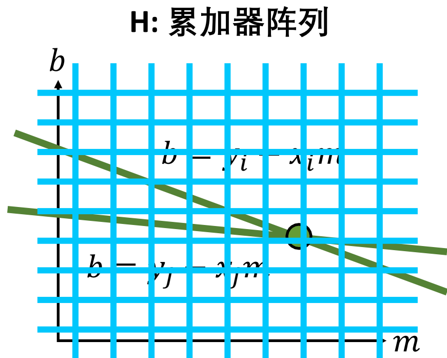
Hough (参数) 空间
